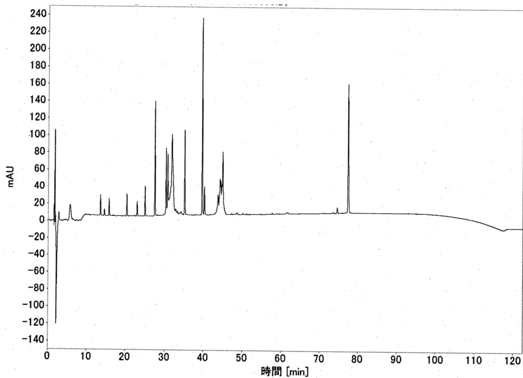
図1 日本薬局方エポエチンアルファ標準品 (Lot EPOa04A) の 確認試験 (2) ペプチドマップにおけるクロマトグラム
